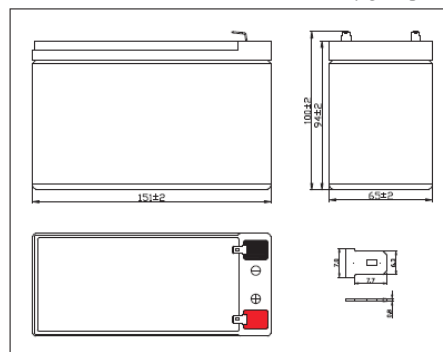
Клеммы F2
