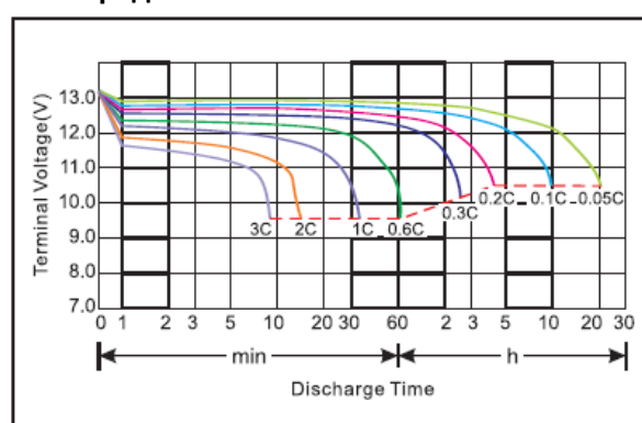
Разрядный ток 25°C
